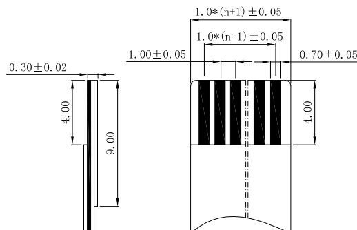
适用电缆
